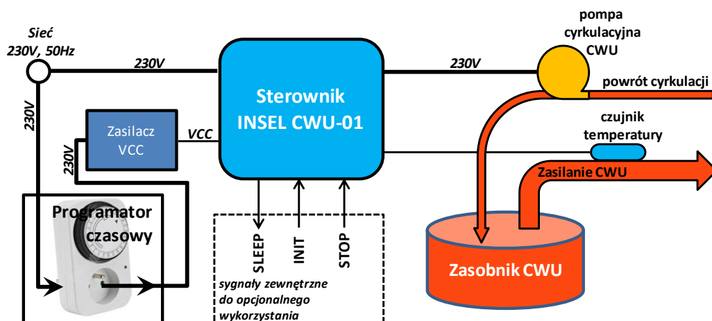
Rys. 4. Podłączenie sterownika do programatora czasowego.
